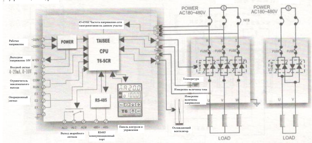
Принципиальная схема управляющего модуля
