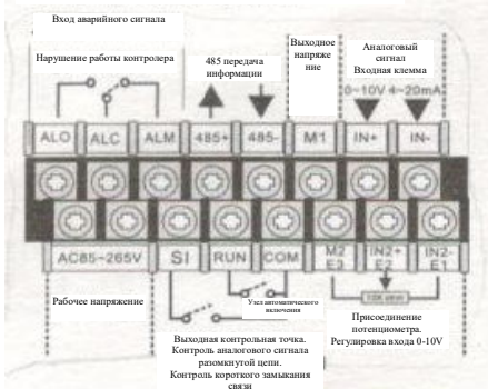
Схема подключения однофазной модели Т6
